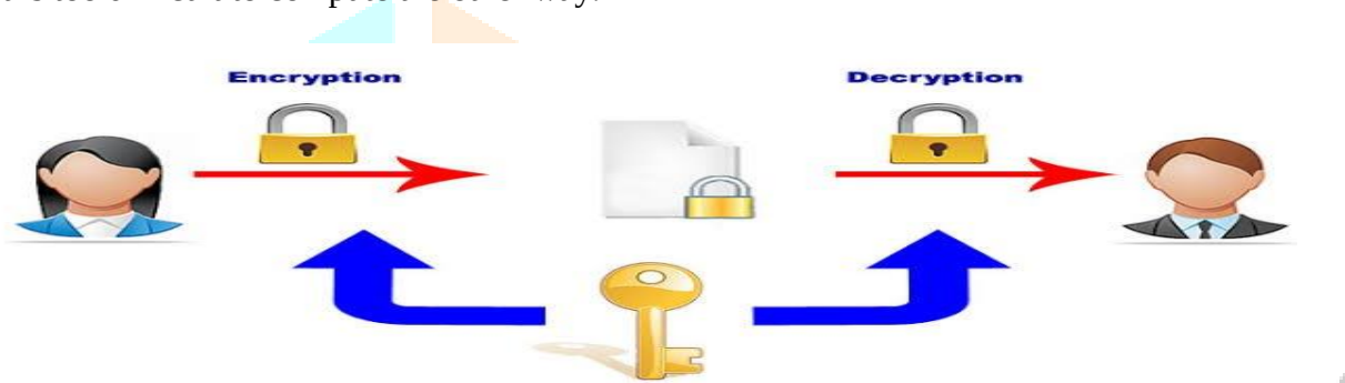
Figure1. Cryptosystem
